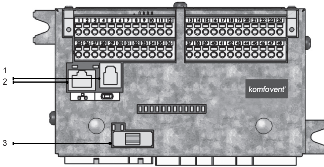
Рис 1.3 а. Контроллер с клеммами для подключения
